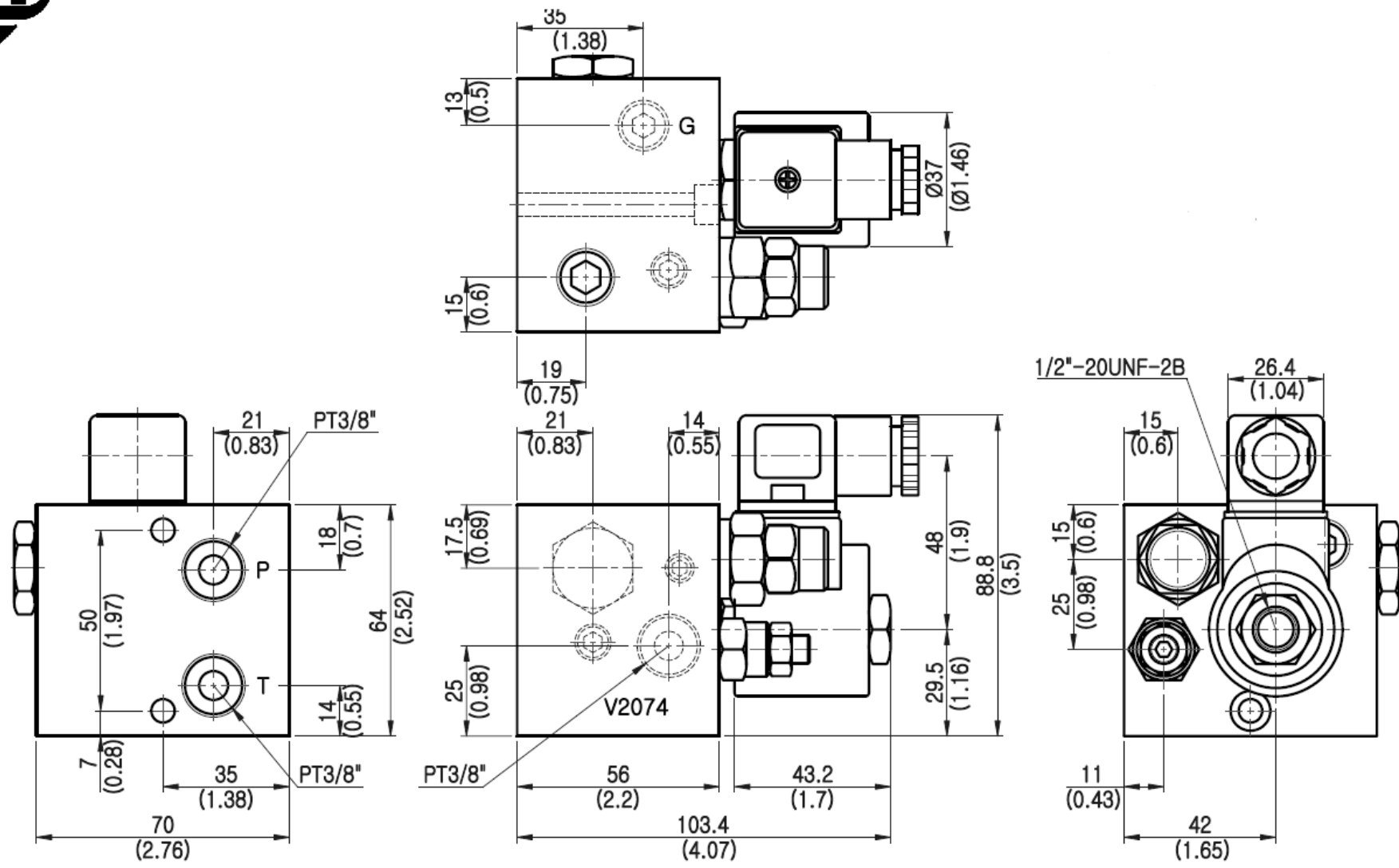
MODEL: SV-2074 單位:mm Unit:mm
